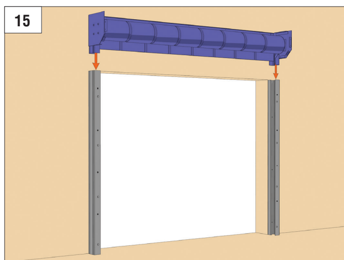
15 Установите короб с противопожарной шторой сверху направляющих (рис. 15, 16).
