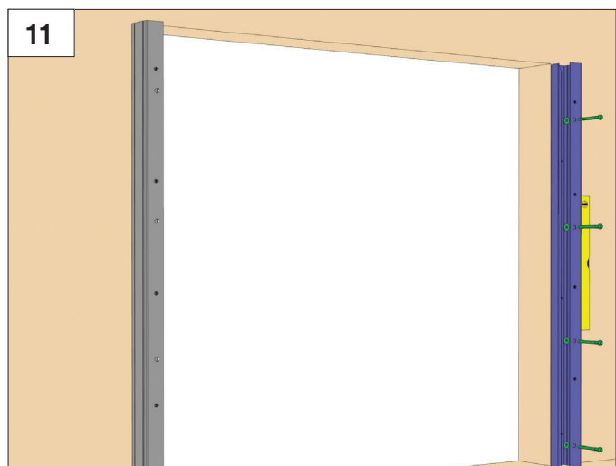
11 Установите и закрепите противоположную направляющую в проеме.
