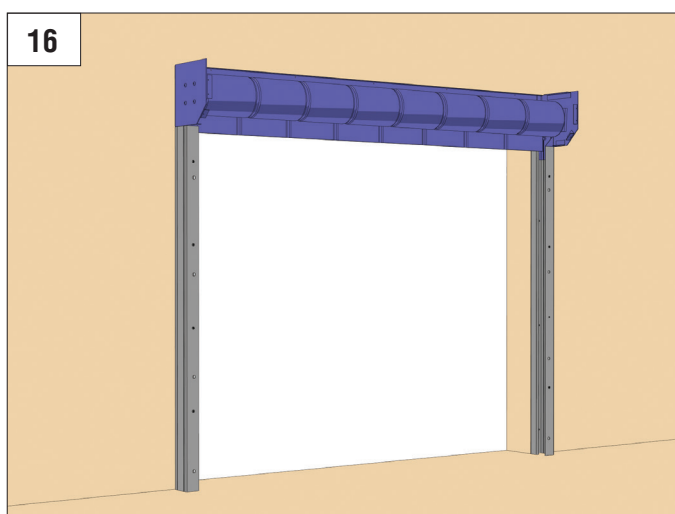
15 Установите короб с противопожарной шторой сверху направляющих (рис. 15, 16).
