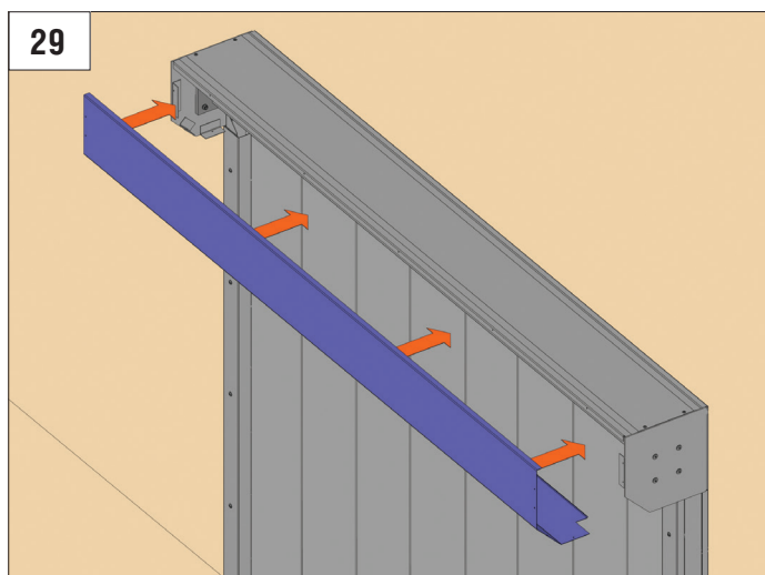
Установите переднюю крышку короба.
