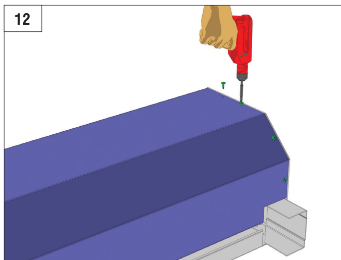
12 Снимите переднюю крышку короба.
