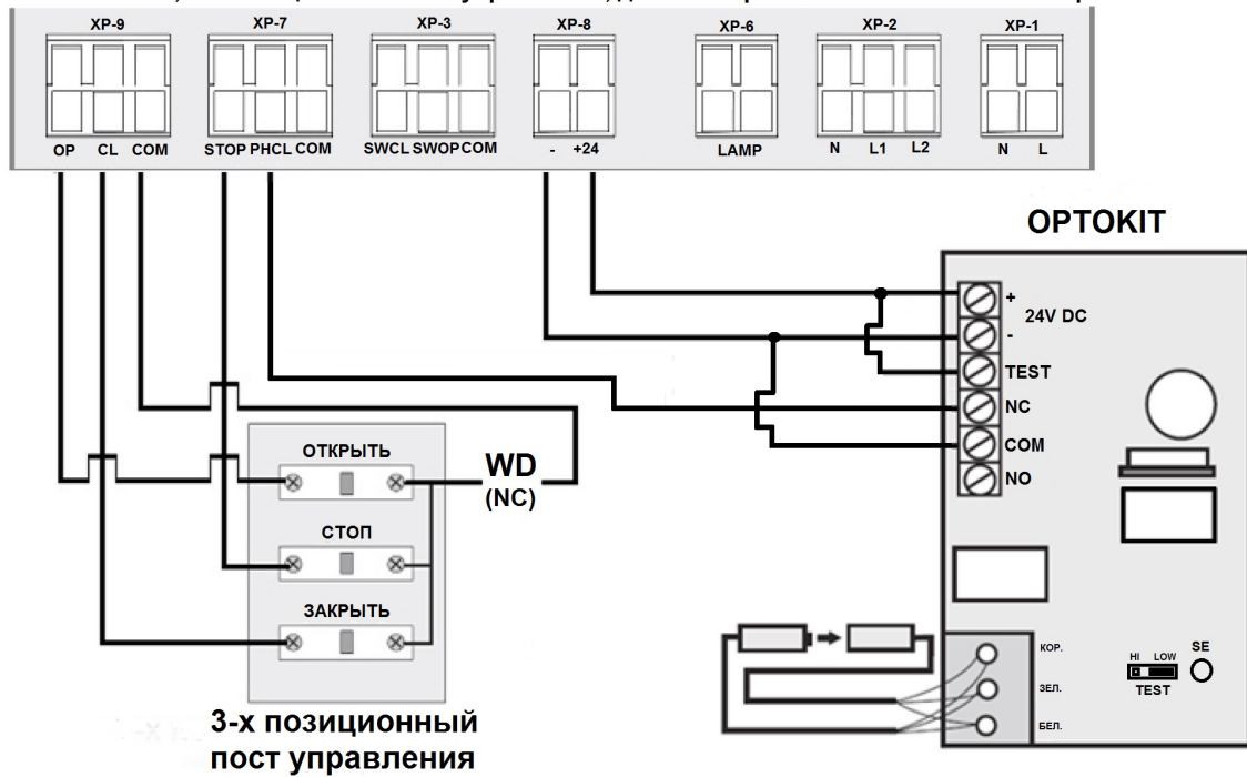
Схема РСВ-SH, 3-х позиционный пост управления, датчик открытой калитки и оптосенсоры
